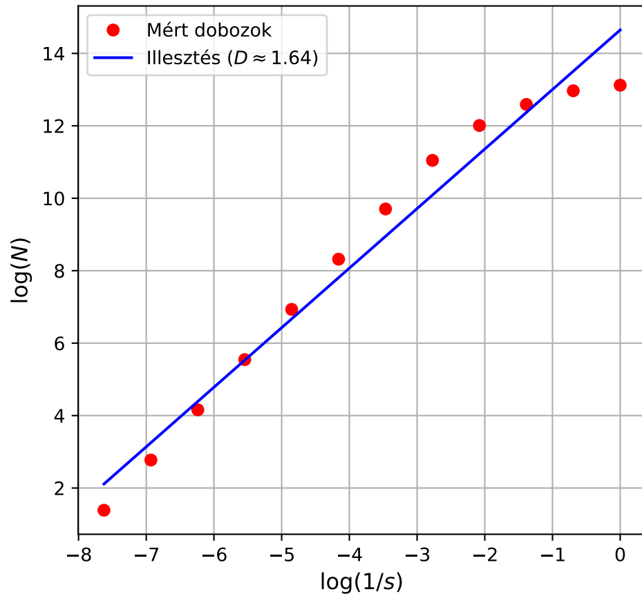
Erdős-tűz modell
